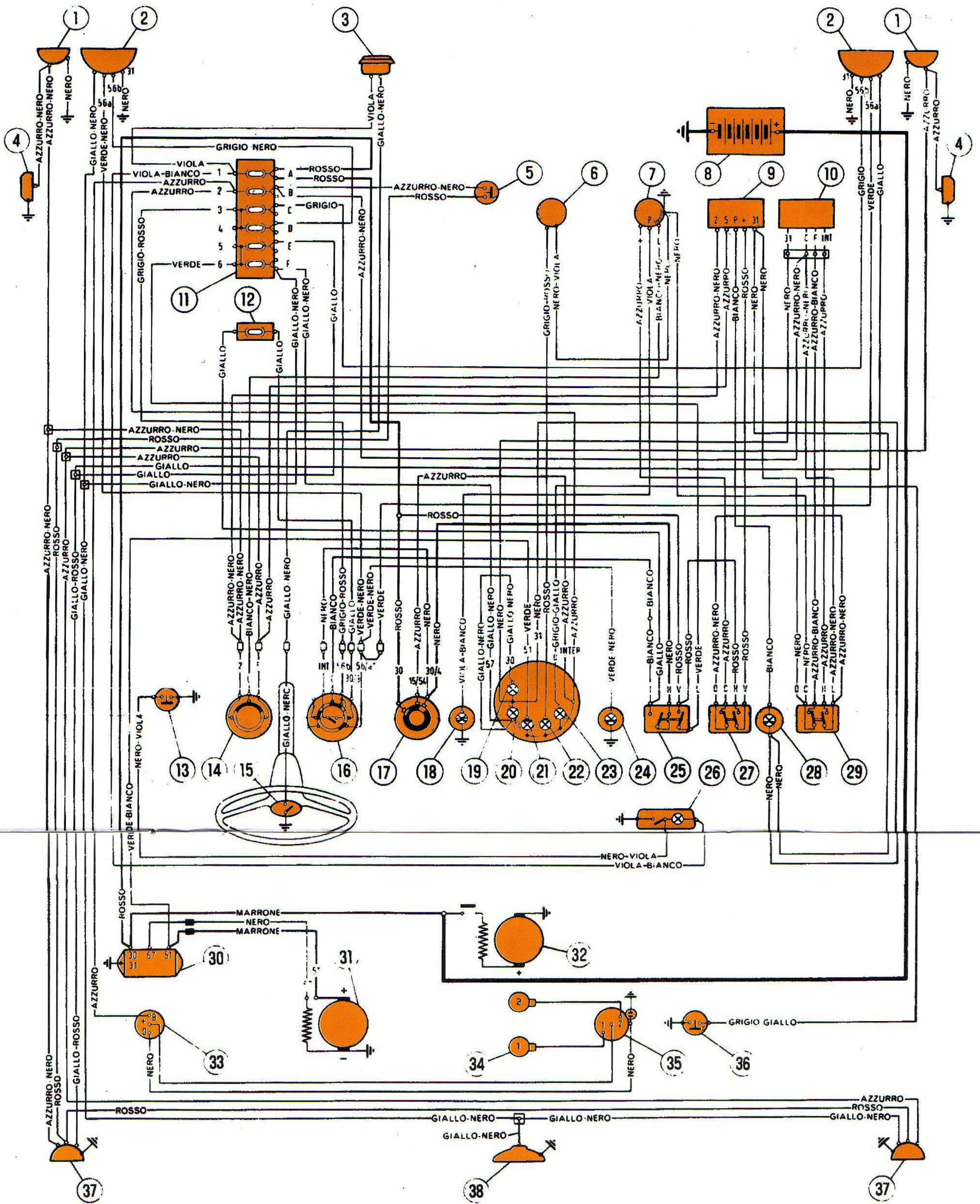
SCHALTPLAN DER ELEKTRISCHEN ANLAGE
